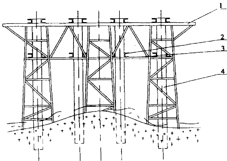
图 B.0.8 支撑式钢桁架平台结构示意图
