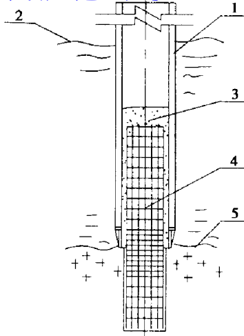
图 B.0.3 预制型芯柱嵌岩桩嵌岩型式示意图
