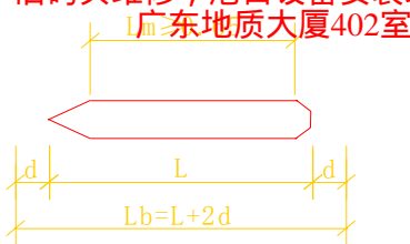
图 4.3.1-1 单个泊位长度与码头长度
