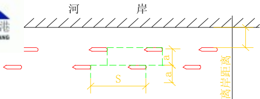
图 A. 1. 1 抛锚系泊锚位
