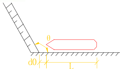
图 4.3.3 直立式码头与斜坡护岸相接处布置
